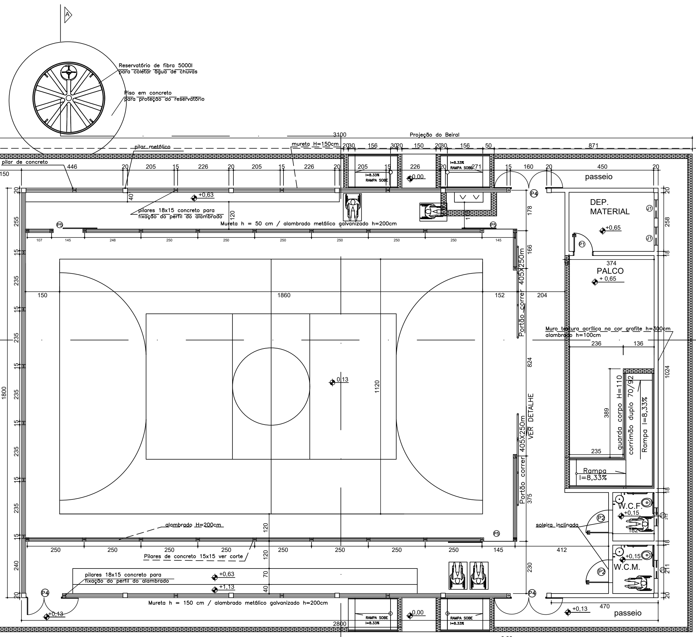
PLANTA QUADRA COBERTA 504,00 m2 Escala 1/100 OBS: As demarcações a serem executadas no piso não correspondem as medidas oficiais.
